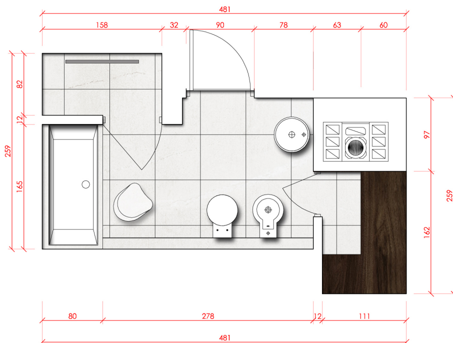
rzut/1:50
